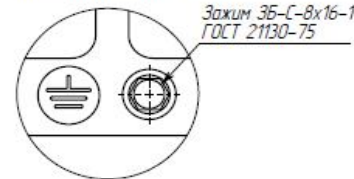
Б Заземление насоса
