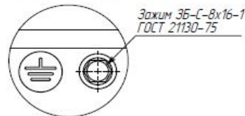
А Заземление рамы агрегата
