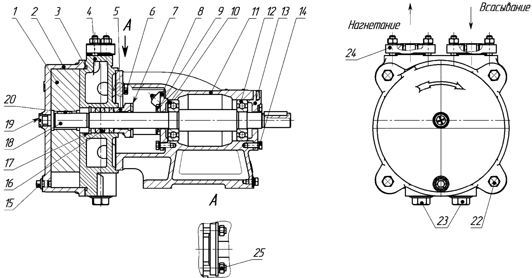
Рисунок 2 – Разрез насоса
