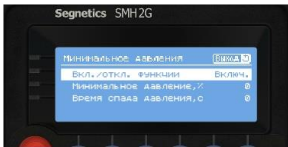
Рисунок 11. Минимальное давление
