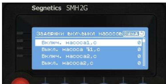
Рисунок 16. Задержки включения/выключения насосов
