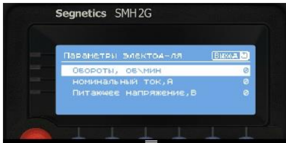
Рисунок 9. Параметры электродвигателя
