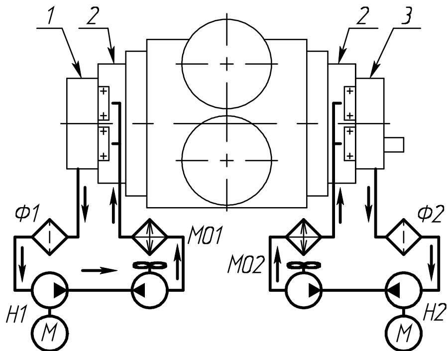
Рисунок 5 – Схема смазки подшипников насоса Φ – фильтр; Н – маслонасос; МО – маслоохладитель; 1 – крышка задняя; 2 - корпус подшипника; 3 – крышка редуктора.
